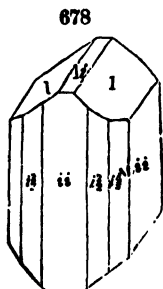
Schneeberg.
